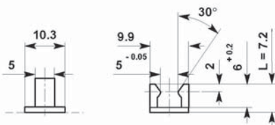
Spindle type 12 Optional
