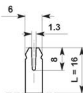
Spindle type 8 Optional
