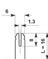
Spindle type 8 Optional
